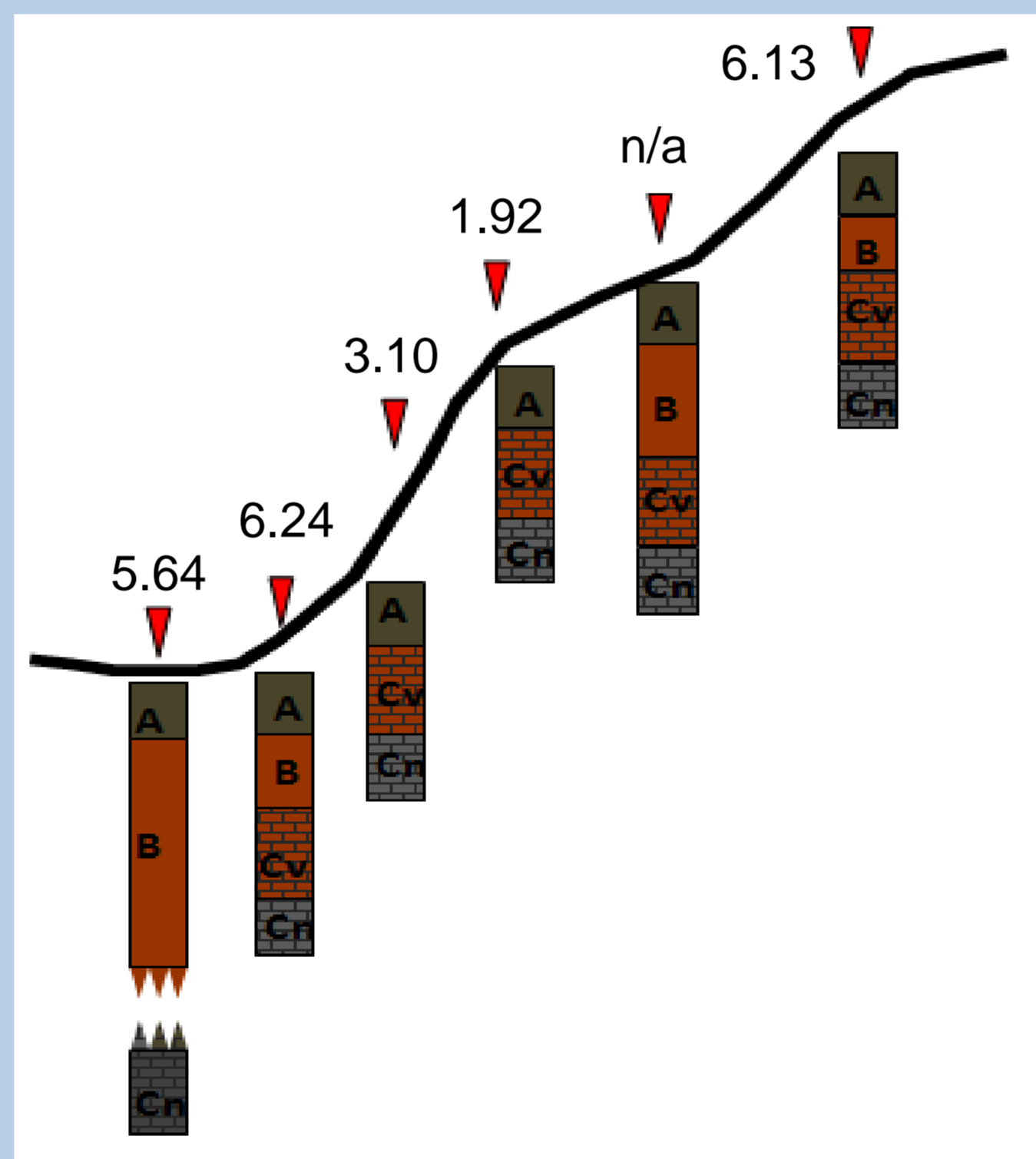
Abb.2: Schematische Horizontabfolge des untersuchten Hanges mit der gemessenen CO 2 -Konzentration in µg CO 2 / h * g
